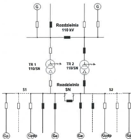
Rys.2. Konfiguracja minimalna GPZ
