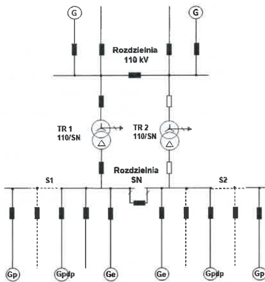
Rys.1. Konfiguracja maksymalna GPZ
